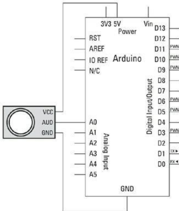
FIGURE 12-15 Schéma du circuit d'un microphone électret.
