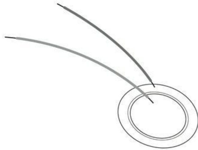
FIGURE 8-15 Un buzzer piézo en dehors de sa coquille.
