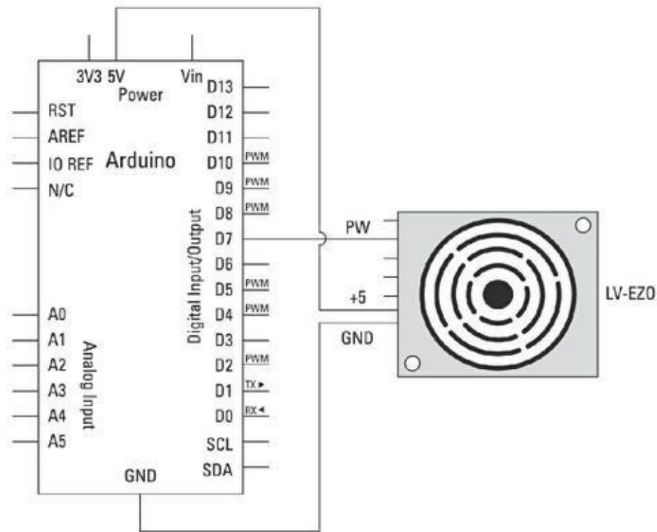
FIGURE 12-14 Schéma de principe exploitant un LV-EZO.
