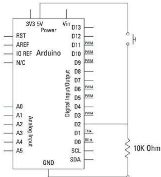
FIGURE 11-5 Le schéma de câblage du circuit StateChangeDetection.
