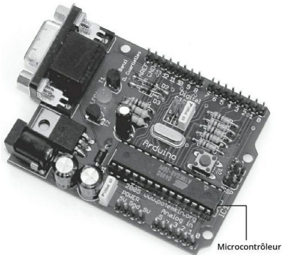
FIGURE 1-3 La carte série Arduino originelle.
