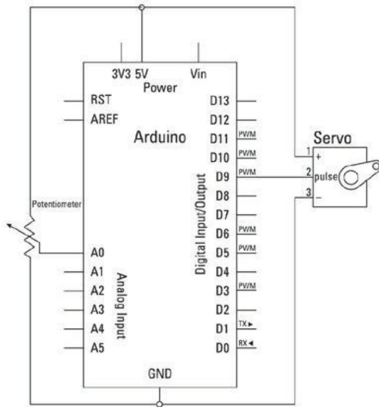
FIGURE 8-12 : Un circuit de servomoteur piloté par un potentiomètre.
