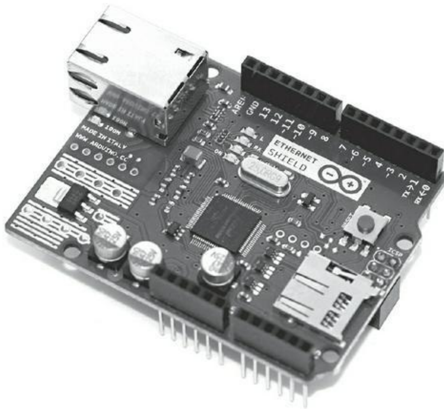
FIGURE 13-7 Une carte fille Ethernet (sans le module PoE).
