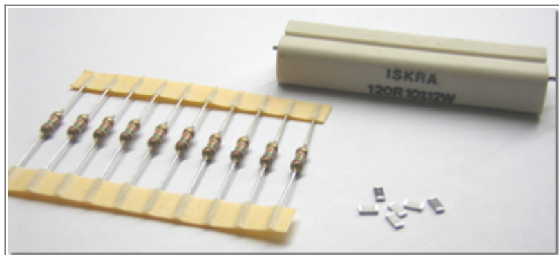
A gauche des résistances carbone 1/4W, à droite des résistances CMS, en haut une résistance de puissance 12W
