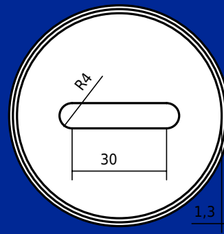
Vue dessous
